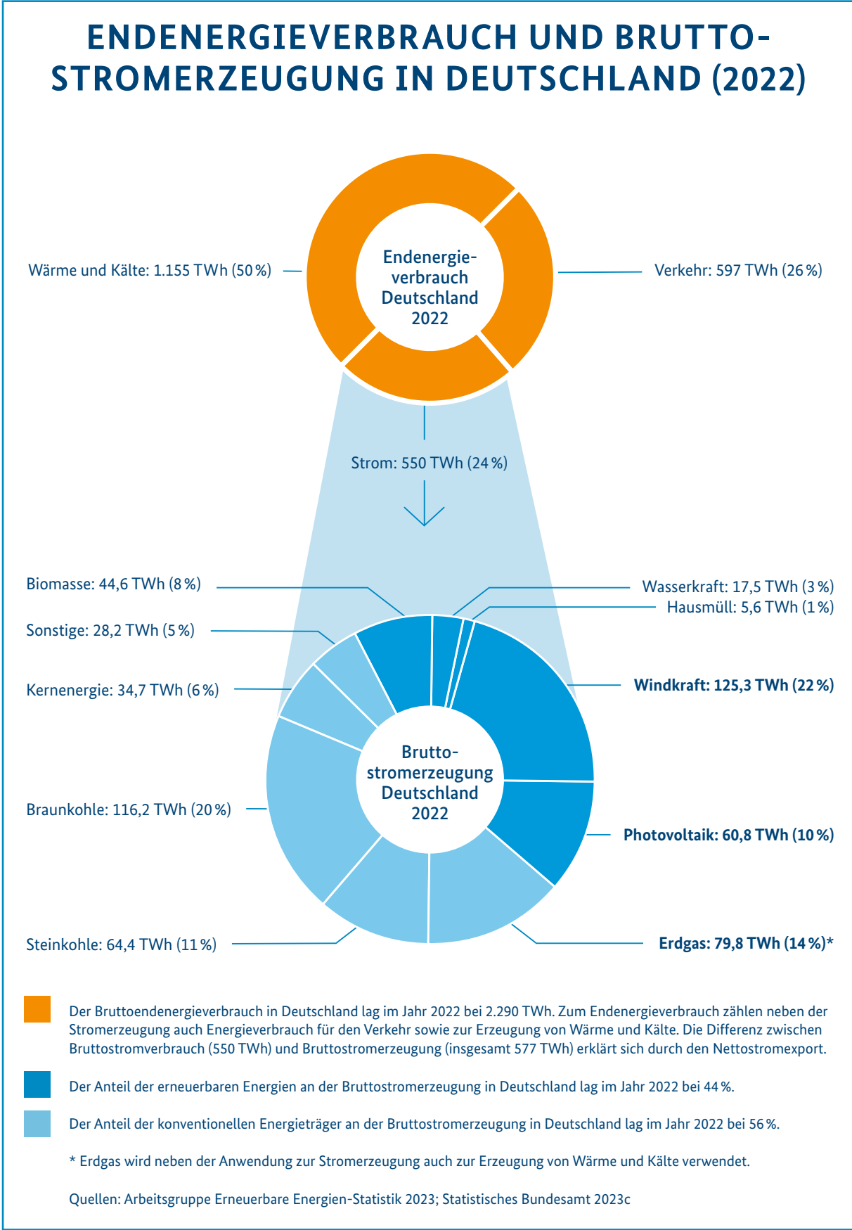
Abbildung 1: Endenergieverbrauch und Bruttostromerzeugung in Deutschland (2022) Quelle: UBA 2023a
